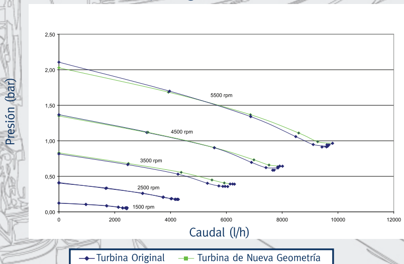
Performance comparativa de turbinas de bomba R-129 (Original) vs Diseño Dolz
